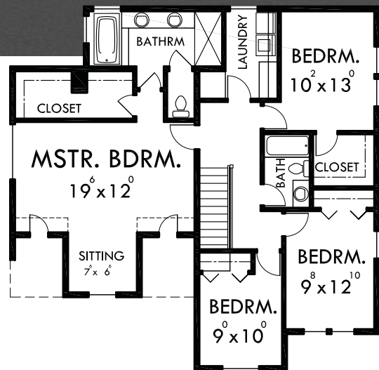
UPPER FLR.
